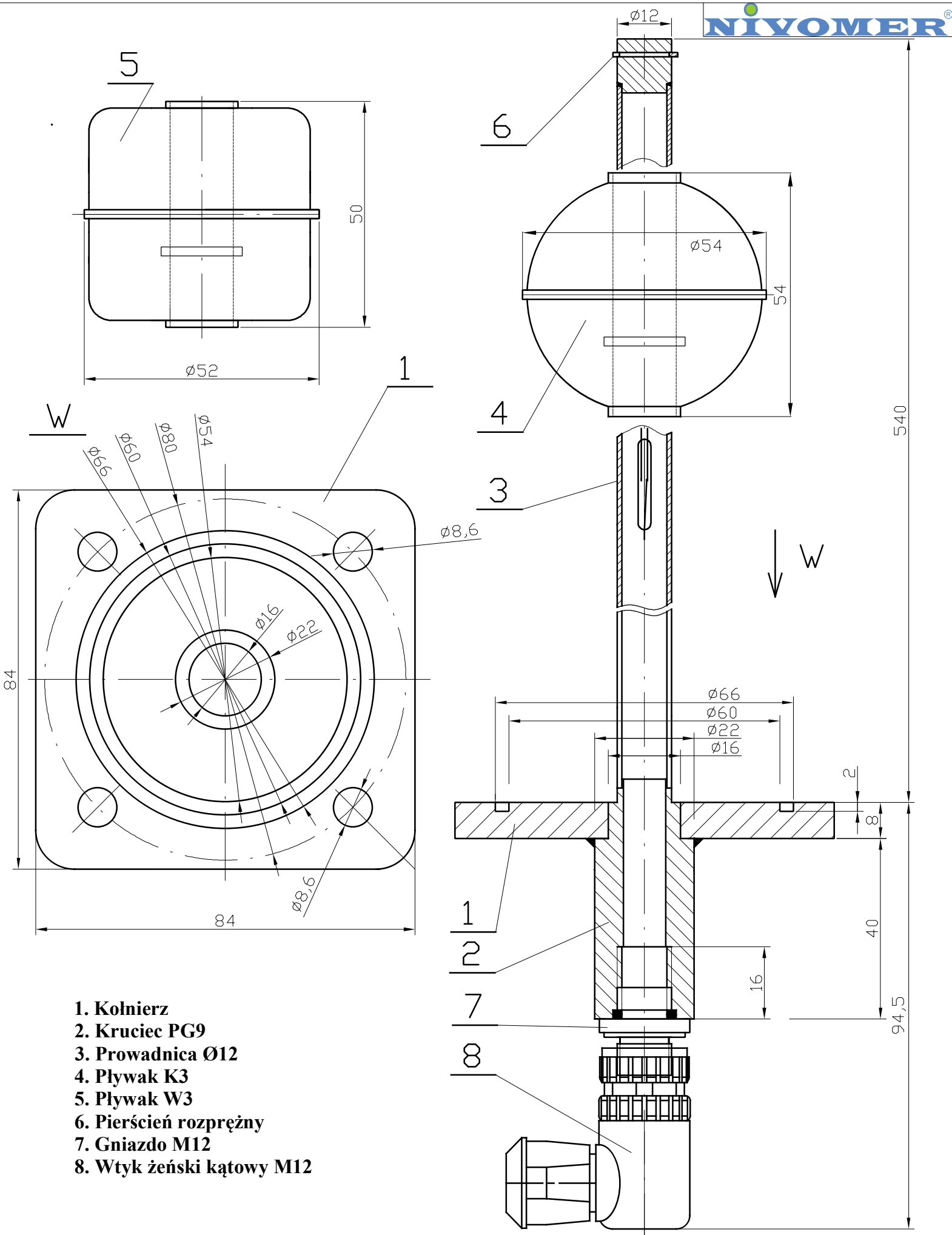
Rys. RT-2. Miernik pływakowy CP-1 z przyłączem kołnierzowym
