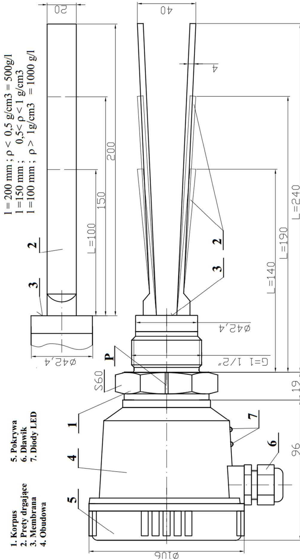
Rys.7. Wibracyjny sygnalizator poziomu WSP-1A
