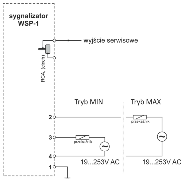
Rys. 6. Podłączenie sygnalizatorów WSP-1/A z wyjściem bezkontaktowy przełącznik elektroniczny.
