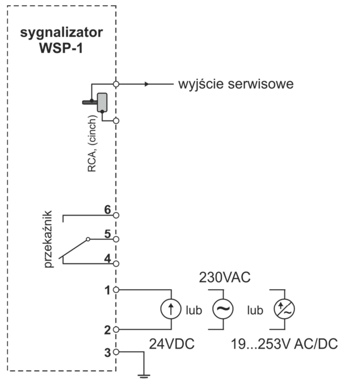
Rys. 4. Podłączenie sygnalizatorów WSP-1/A.
