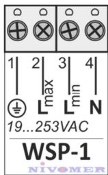
Rys. 5. Podłączenie sygnalizatorów WSP-1/A dla wyjścia typu bezkontaktowy przełącznik elektroniczny
