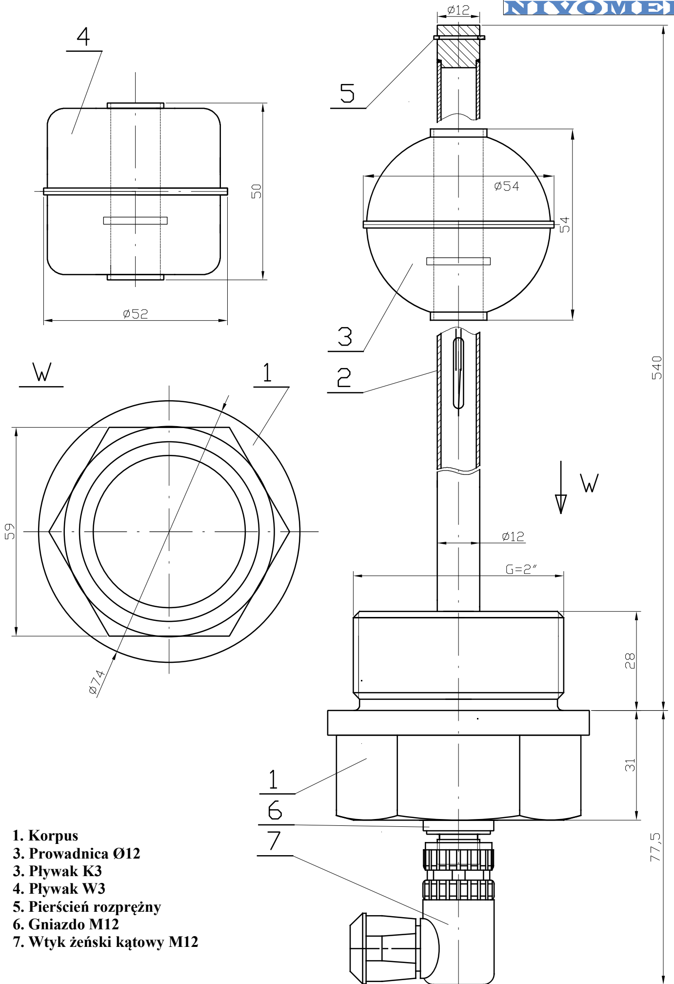
Rys. RT-1. Miernik pływakowy CP-1 z przyłączem G=2"
